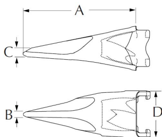
Ząb płaski komplet ESCO17
