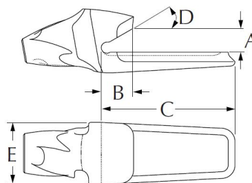
Ząb płaski ESCO17
