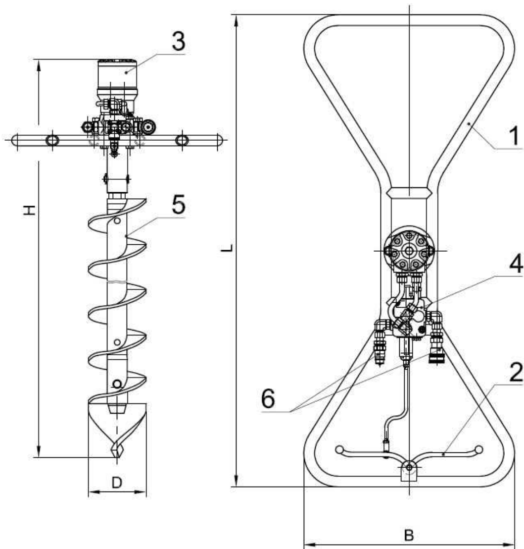
RĘCZNA WIERTNICA PIONOWA TYPU RWP-150
